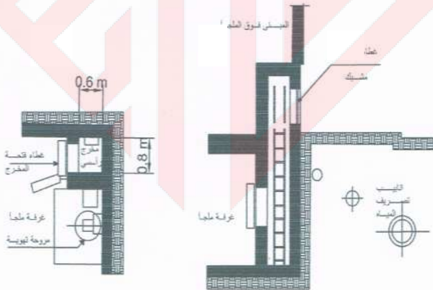
الشكل 6/3-5: مخرج رأسي للملجأ مع انابيب تصريف مياه المجاري [2]
