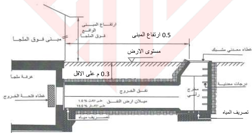
الشكل 5-3/10: نفق ينتهي بمخرج رأسى [2]
