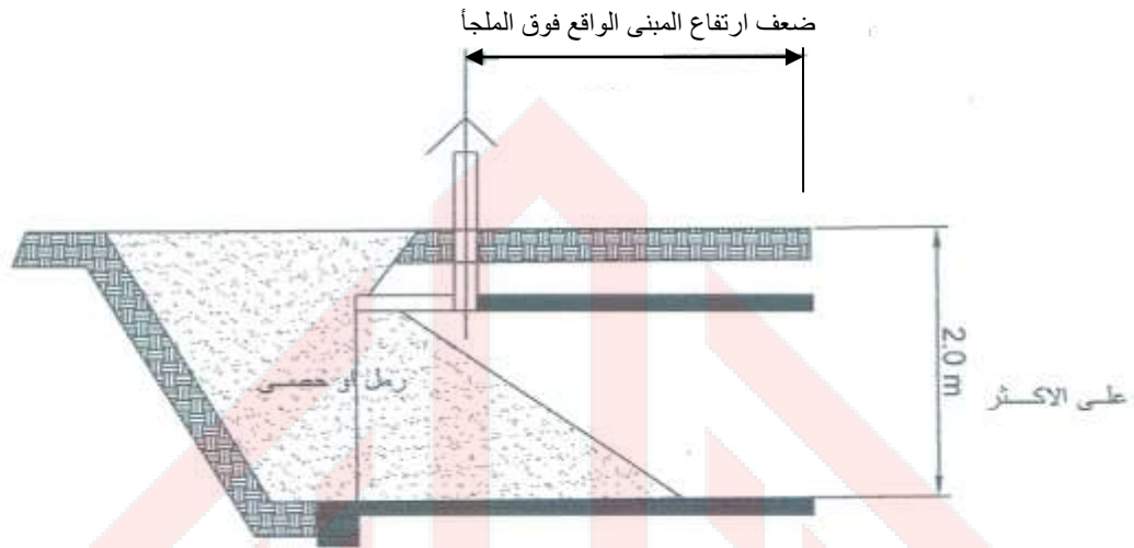
الشكل 5-11/3: نفق ذو نهاية مطمورة [2]
