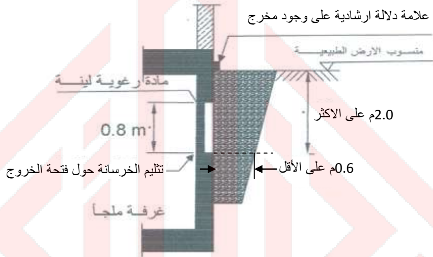
الشكل 5-9/3: مخرج رأسي مدفون [2]
