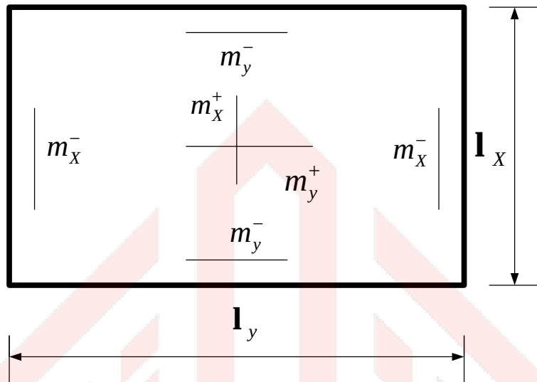
الشكل 6-2/5: العزوم في البلاطات ذات الاتجاهين
