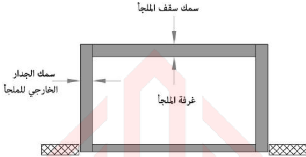
الشكل 6-1/4: أقل سمك مسموح به لسقف الملجأ وجدرانه الخارجية [1]
