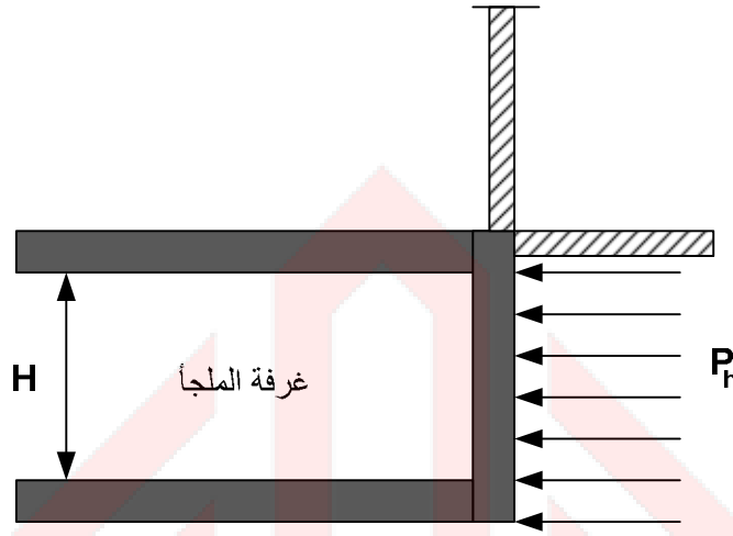
الشكل 6-9/4: الاحمال المؤثرة على جدار ملجأ مظمور كلياً بالتربة[1]
