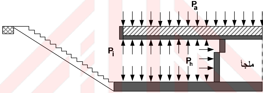
الشكل 6-14/4: أحمال الممرات المحصنة المؤدية إلى الخارج [1]
