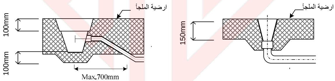
الشكل 8-4/1: التصريف الارضي في ارضية الملجأ[1]
