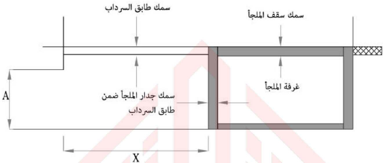
الشكل 6-4/4: أقل سمك مسموح به لجدران الملجأ المشيد ضمن الطابق [1]
