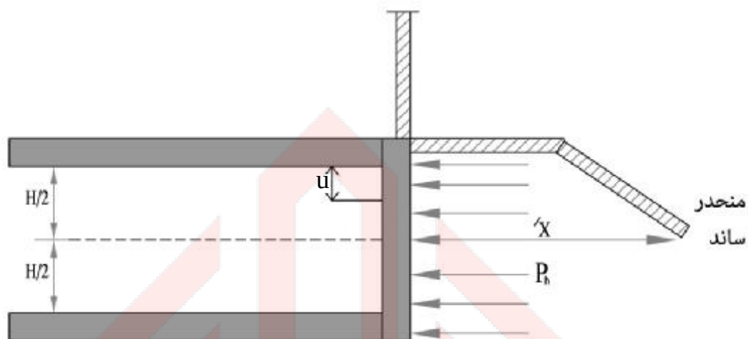
الشكل 6-11/4: الاحمال المؤثرة على جدار ملجأ مطمور كلياً بالتربة من منحدر او جدار سائد[1]
