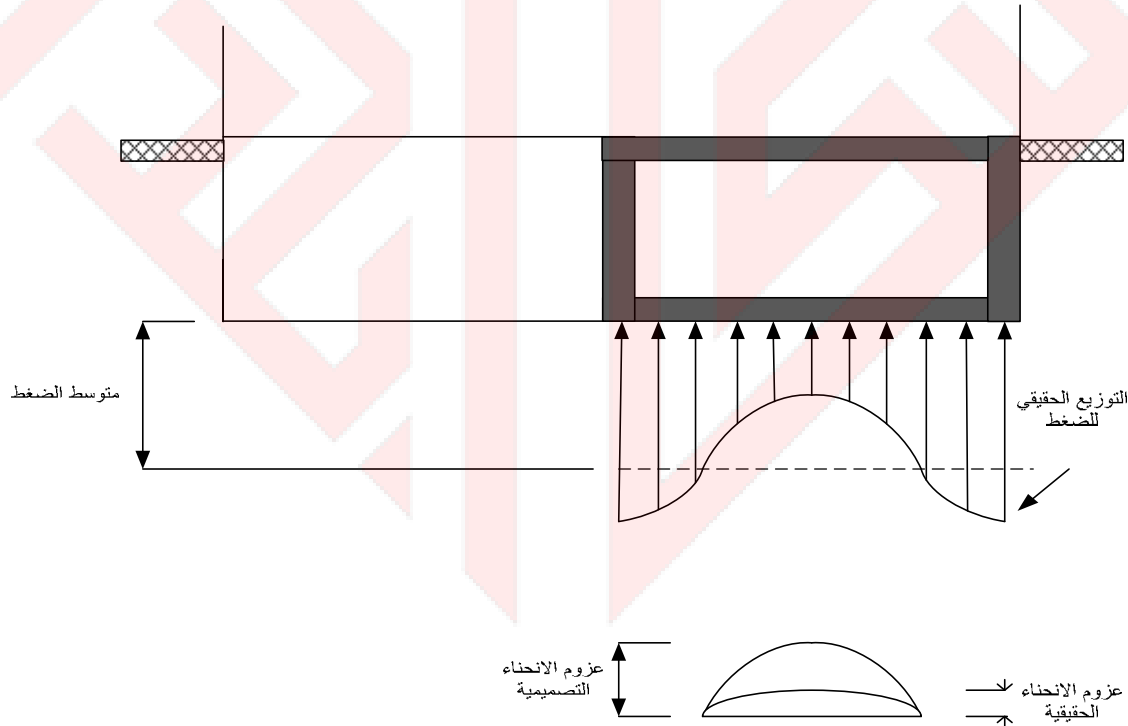
الشكل 6-7/4: توزيع ضغط التربة تحت أرضية الملجأ [1]
