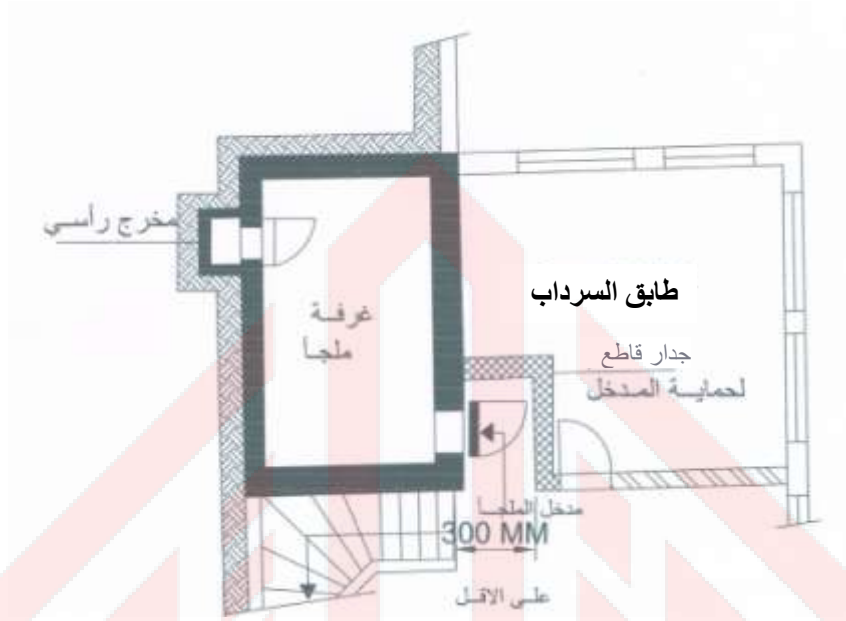
الشكل 5-2/1: حماية باب الملجأ من الاشعاعات وموجات العصف المباشر [2]
