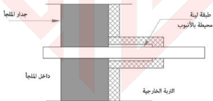
الشكل 8-2/1: حماية الاتابيب المدفونة في التربة والتي تخترق هيكل الملجأ [1]
