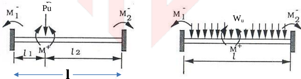
الشكل 1/5-6: عزوم الانحناء في العتبات المثبتة
