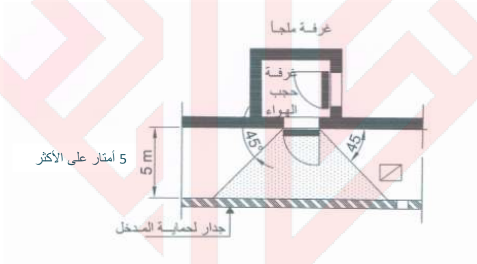
الشكل 5-2/2: زاوية السقوط بين باب الملجأ والجدار الفاصل [2]
