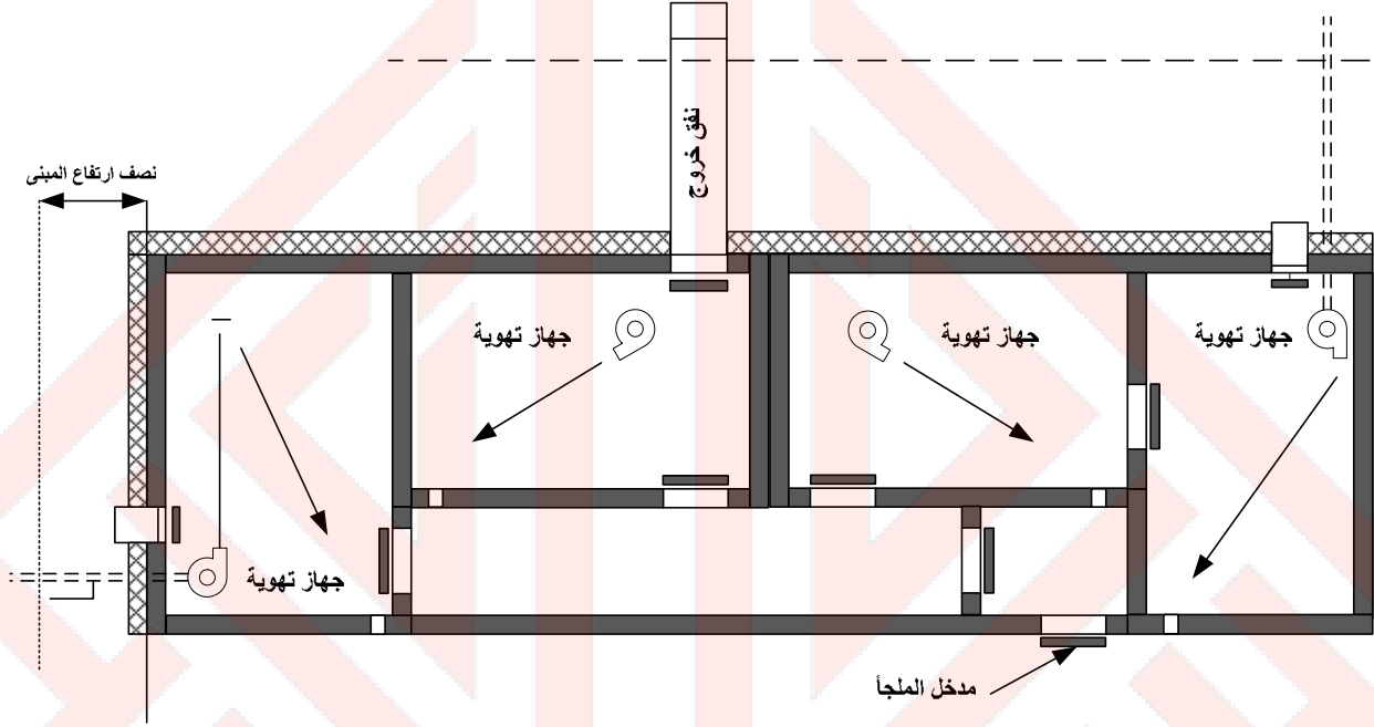
الشكل 7-2/5: تجهيز الهواء لغرفتي ملجأ من خلال فتحة مشتركة[1]
