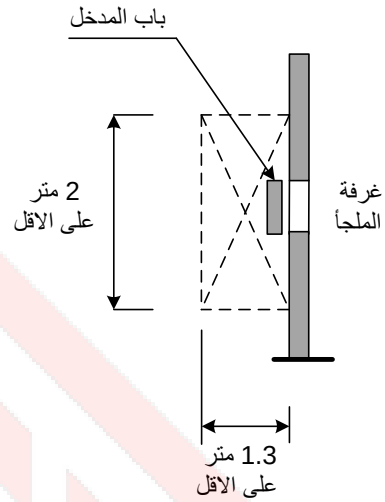
(أ) مسقط افقي (4/2-5)
