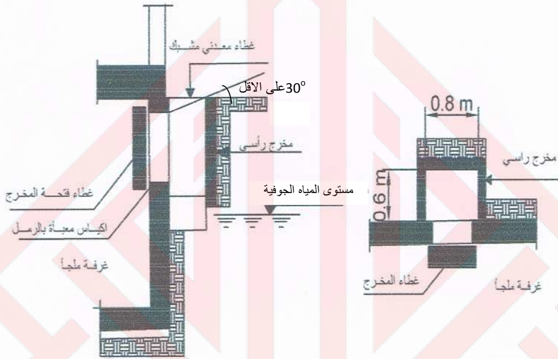
الشكل 5-7/3: مخرج طواريء رأسي مرتفع [2]
