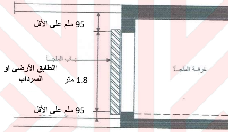
الشكل 5-4/2ب: مقطع شاقولي يبين ارتفاع عتبة المدخل [2]
