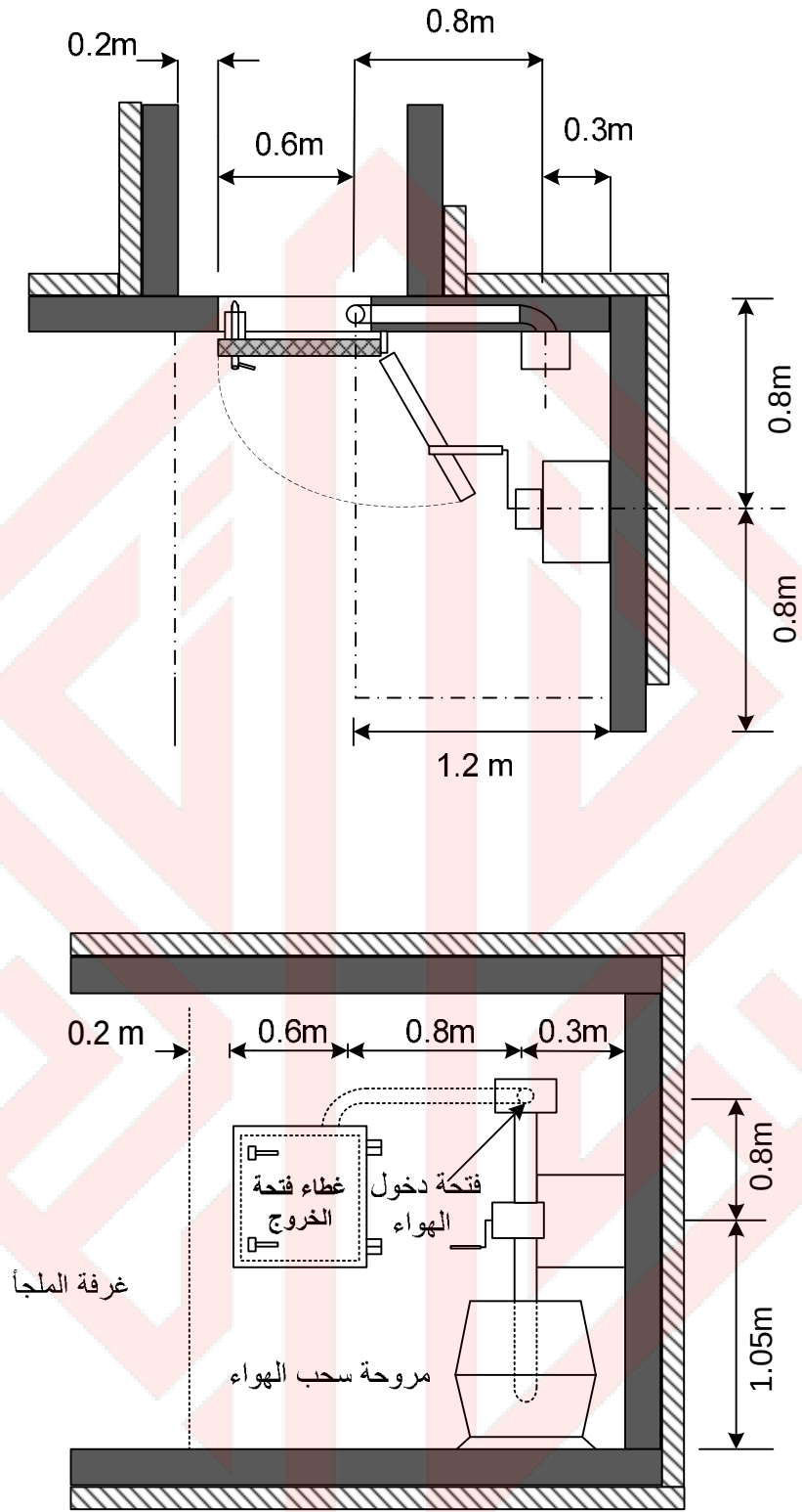
الشكل 7-4/5: مستوى فتحة دخول الهواء [1]
