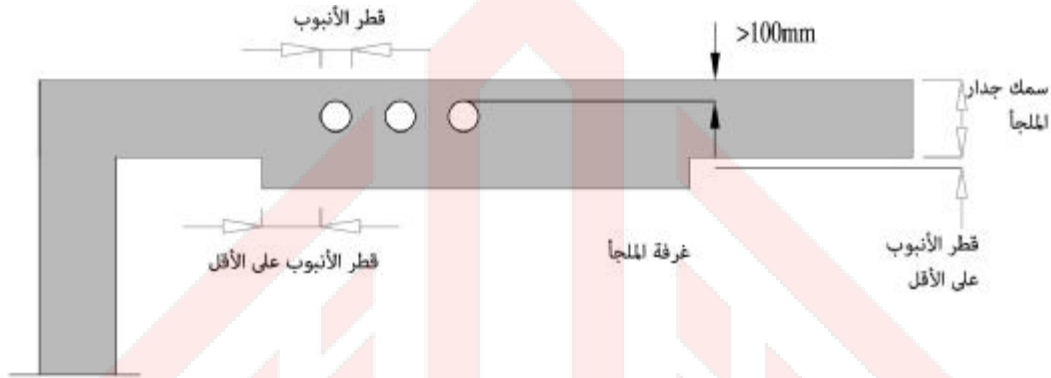
الشكل 5/1-8: توصيلات الانابيب المدفونة في داخل هيكل الملجأ[1]
