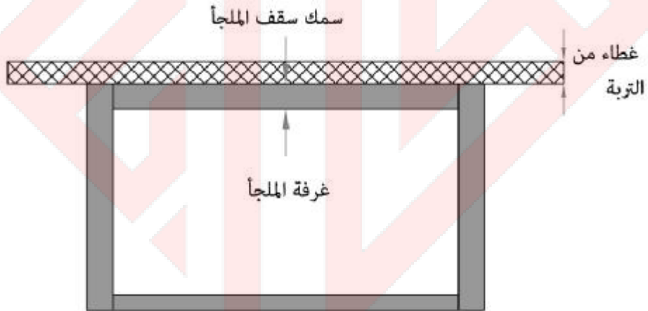
الشكل 6-2/4: أقل سمك مسموح به لسقف الملجأ المغطى بطبقة من التراب [1]
