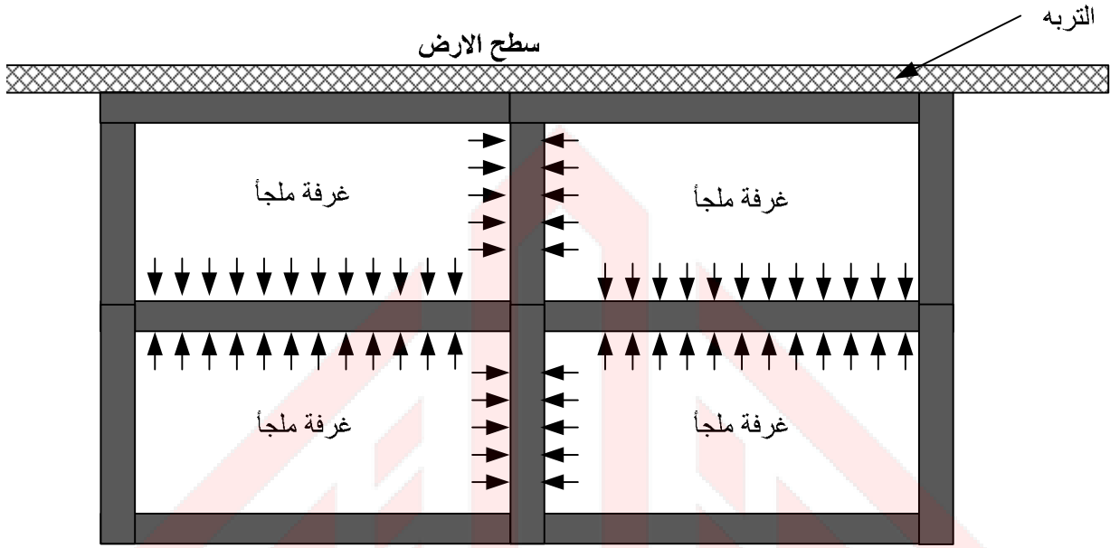
الشكل 6-13/4: مقطع شاقولي يبين أحمال الأرضيات والقواطع الداخلية [1]
