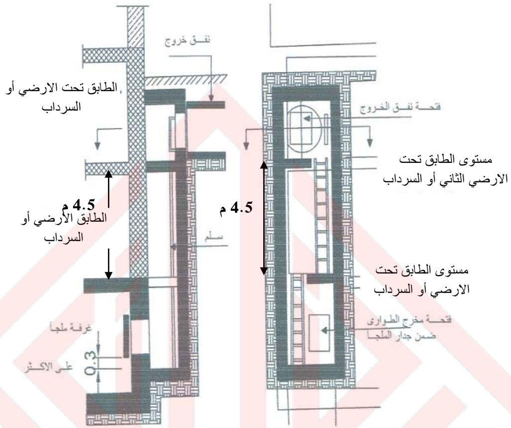
الشكل 5-3/5: مخرج رأسي عميق [2]
