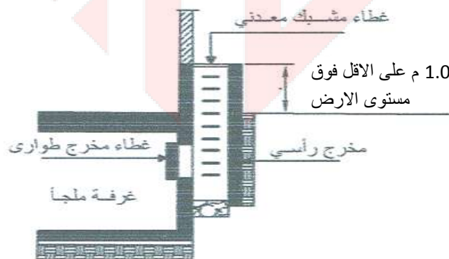
الشكل 5-8/3: مخرج رأسي بالقرب من المناطق المعرضة للفيضانات [2]
