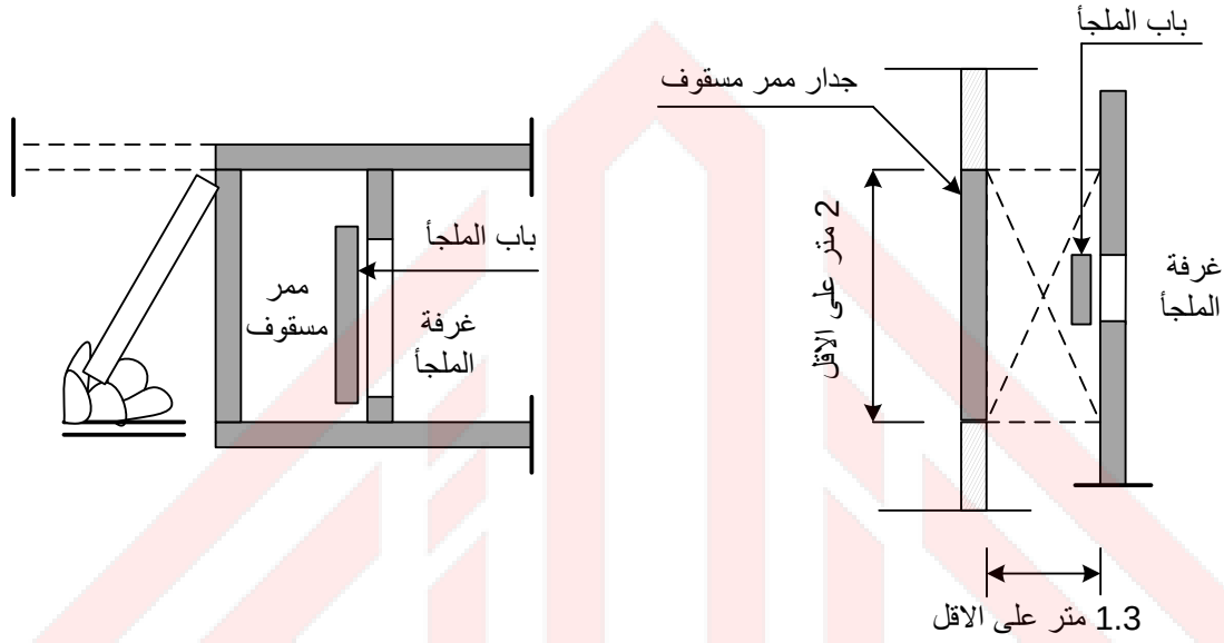
(3/2-5 ب) مسقط شاقولي
