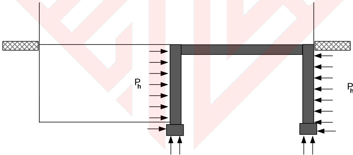
الشكل 6-8/4: الأحمال المؤثرة على جدران الملجأ الخارجية من التربة [1]
