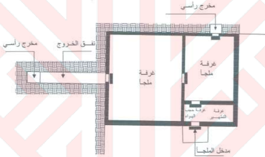
الشكل 5-2 أ: غرفة حجب الهواء وغرفة التطهير [2]
