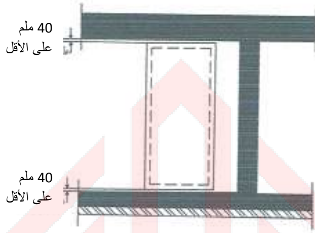
الشكل 5-4/2أ: واجهة مدخل الملجأ [2]
