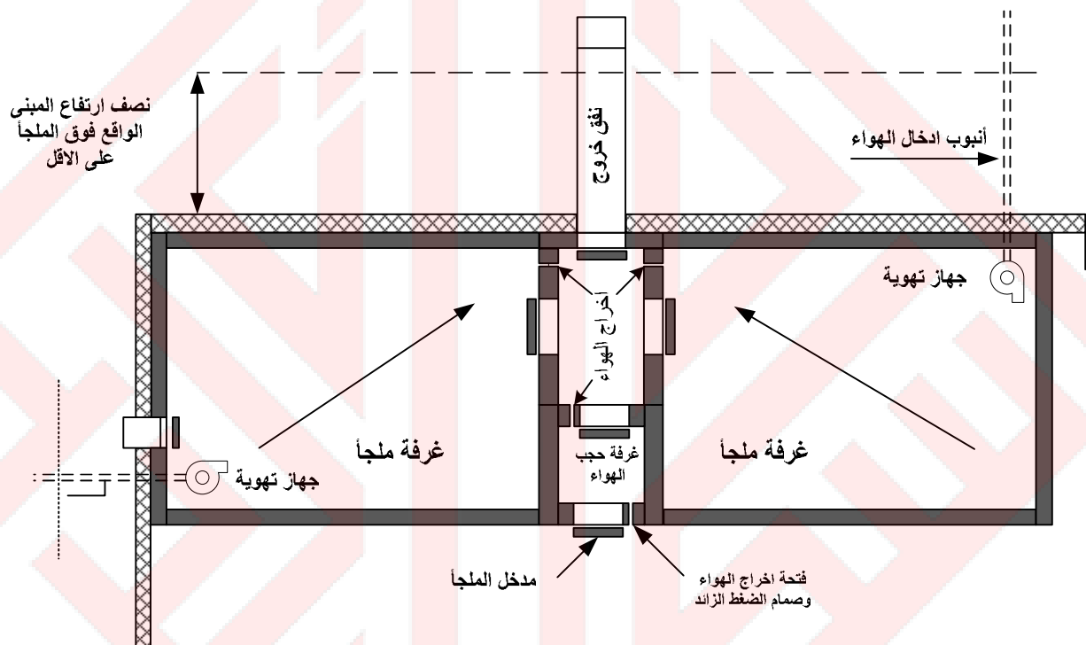
الشكل 7-1/5: تهوية غرف الملجأ [1]
