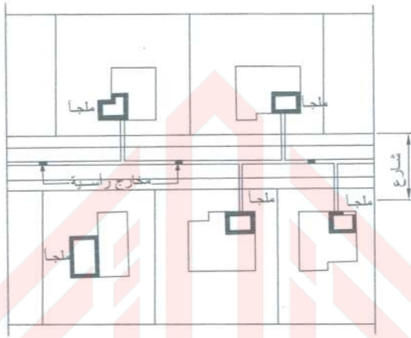
الشكل 5-13: شبكة الانفاق بين المباني المتجاورة [2]
