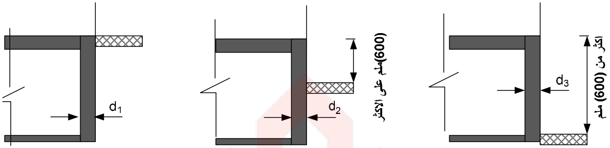
الشكل 6-5/4: أقل سمك مسموح به لجدار الملجأ الملاصق للتربة [1]
