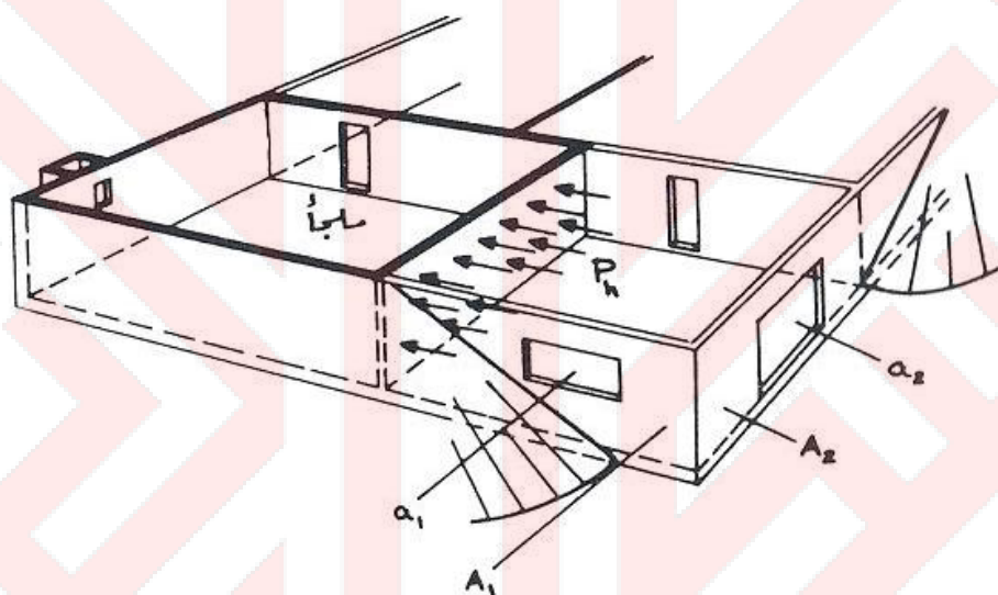
الشكل 6-12/4: ملجأ يقع ضمن الطابق الأرضي أو طابق السرداب [1]
