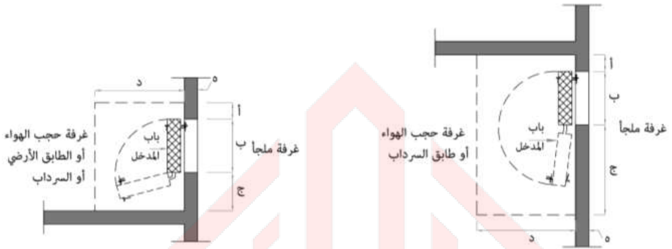
الشكل 5-1/4: الحد الأدنى للمسافات [2]
