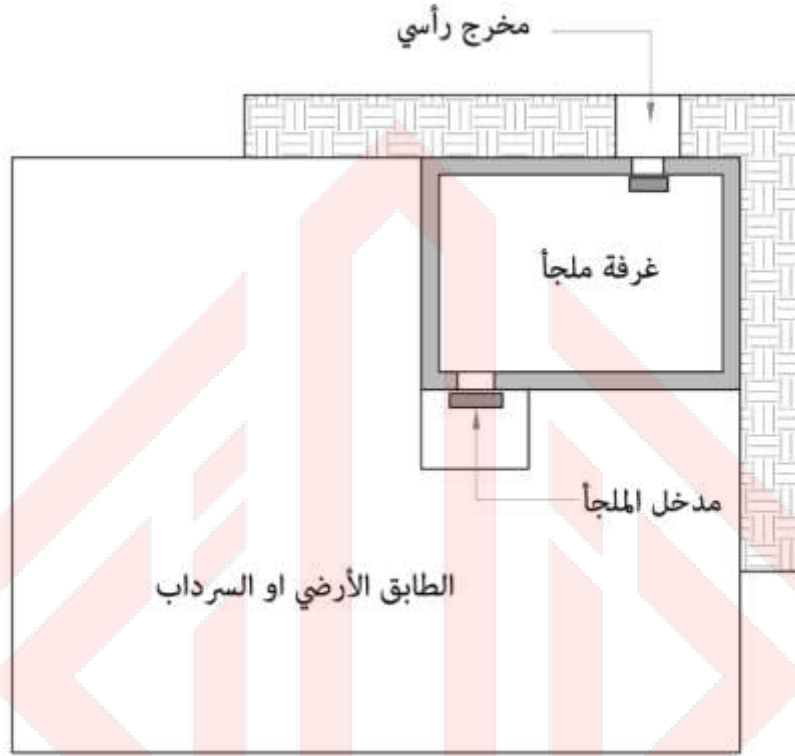
الشكل 5-1: مخارج الطوارئ لملجأ بسعة 13 شخصاً [2]
