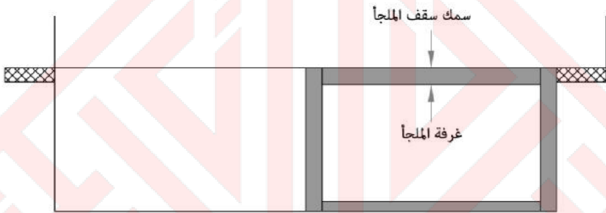
الشكل 6-3/4: أقل سمك مسموح به لسقف الملجأ الواقع تحت مبنى [1]
