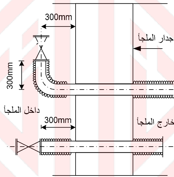
الشكل 8-3/1: صمامات الاغلاق في داخل الملجأ[1]
