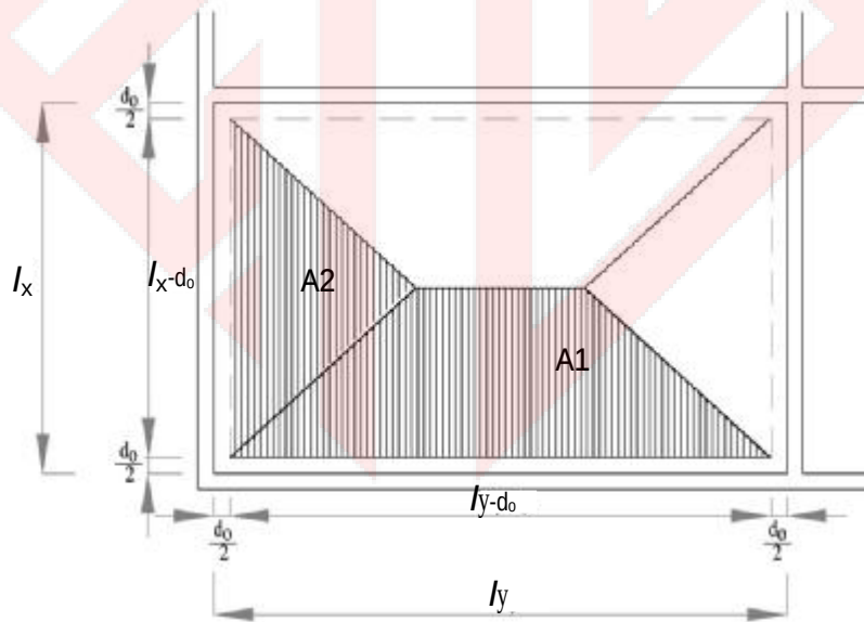
الشكل 6-1/6: خطوط الخضوع ومساحة التحميل في البلاطات (حسابات القص) [1] .
