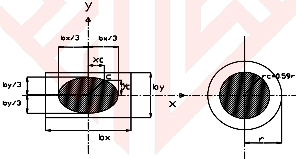
الشكل 2-3/5: موقع تأثير محصلات القوى للأسس المستطيلة والدائرية لتحقيق الأمان من الانقلاب
