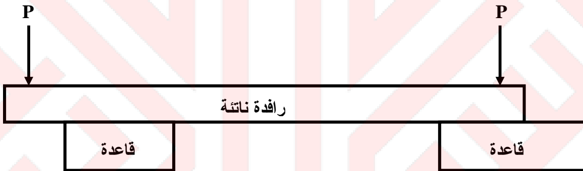
الشكل 3-3/1: أساس نائي
