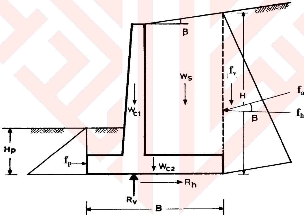
الشكل 5-1/4: القوى المؤثرة على الجدار الساند
