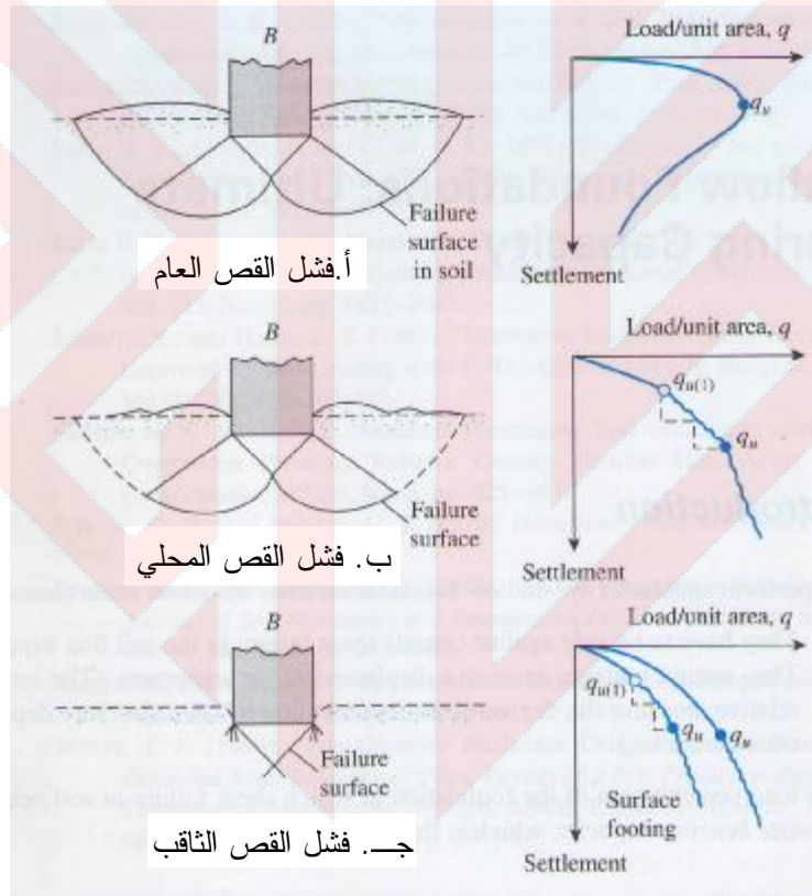
الشكل 3-5/2: تأثير نوع الفشل على قابلية التحمل
