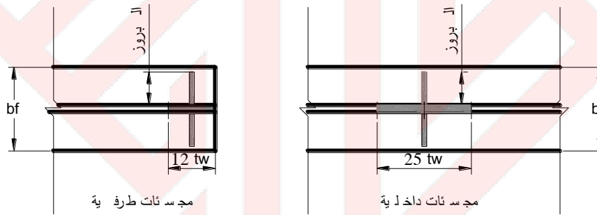
الشكل 11/1-11: مجسئات عرضية (Transverse Stiffeners).
