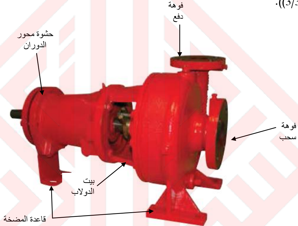
الشكل 6-5/2: مضخة سحب طرفية [6]
