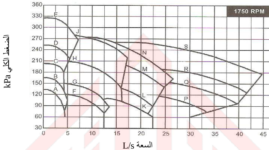
الشكل 6-3/3: منحنيات مصنع نموذجية لمجموعة مضخات [8]
